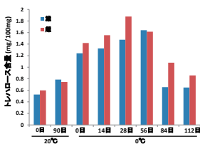
図3 オオタバコガにおける低温による糖の蓄積
