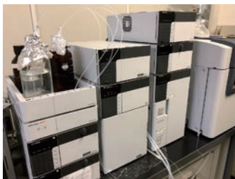
ビタミンB 2 (上)、 液体クロマトグラフィー (下)
