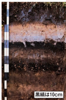
黒ボク土壌の土壌断面
