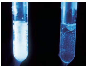
図1 液体の凍結とガラス化
