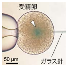
図2 遺伝子導入とGFP蛍光の観察。GFPの情報をもつDNA溶液(矢尻、青緑色)をガラス針で卵に注入(左)。その3日後、幼生の触角でGFPの緑色蛍光を検出(右)。
